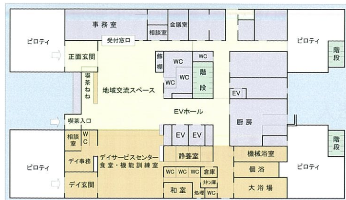
1階平面図
