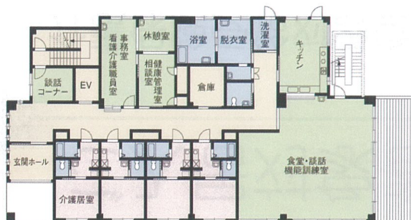
アミーユレジデンス茶屋が坂 平面図 (左:1F 右2.3F)
